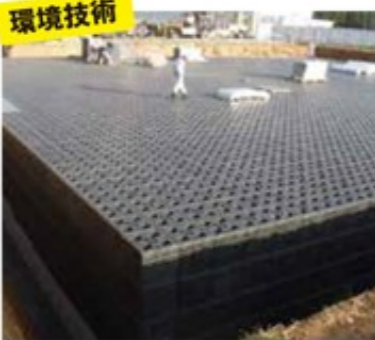
約3,000tの雨水を貯水できる埋設型貯水槽
